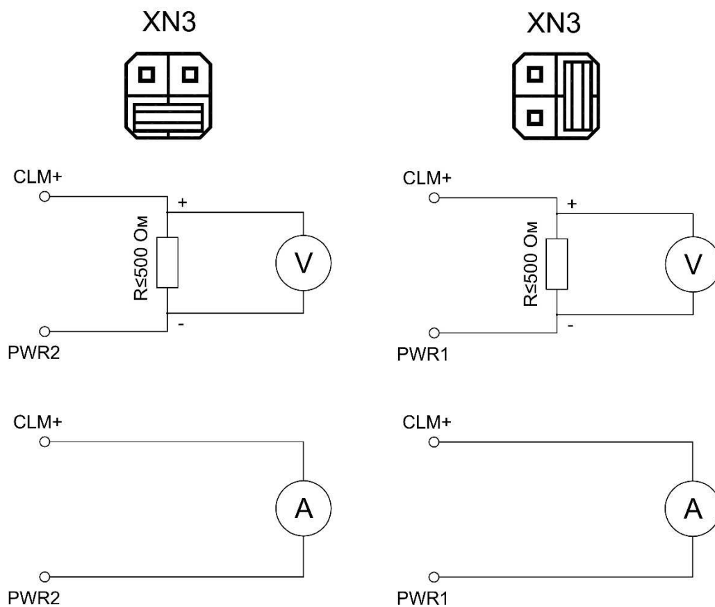
Рисунок Б.2 – Установка перемычки XN3 при подключении по трехпроводной линии: 2 провода питания и один провод CLM+ (активная токовая петля). Заводская установка перемычек: XN3 CLM=PWR2, XN1 RS 485 LOAD disable.
