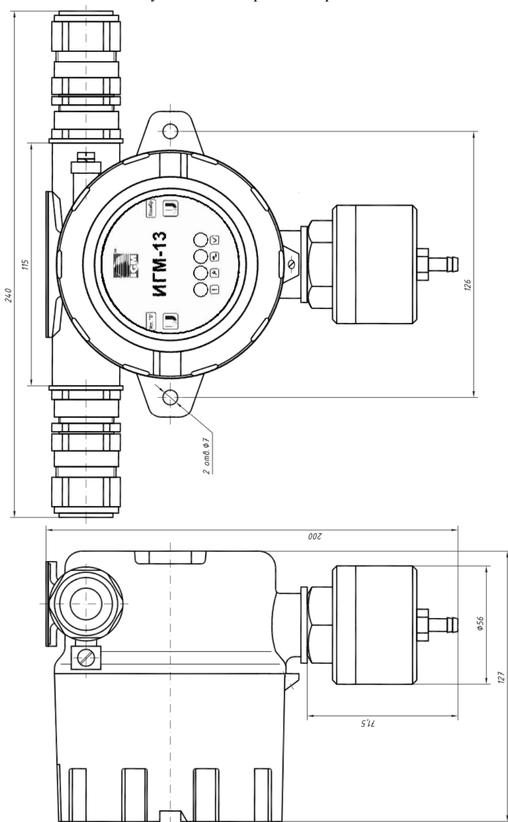
Рисунок Г.1 - Габаритный чертеж ИГМ-13.
