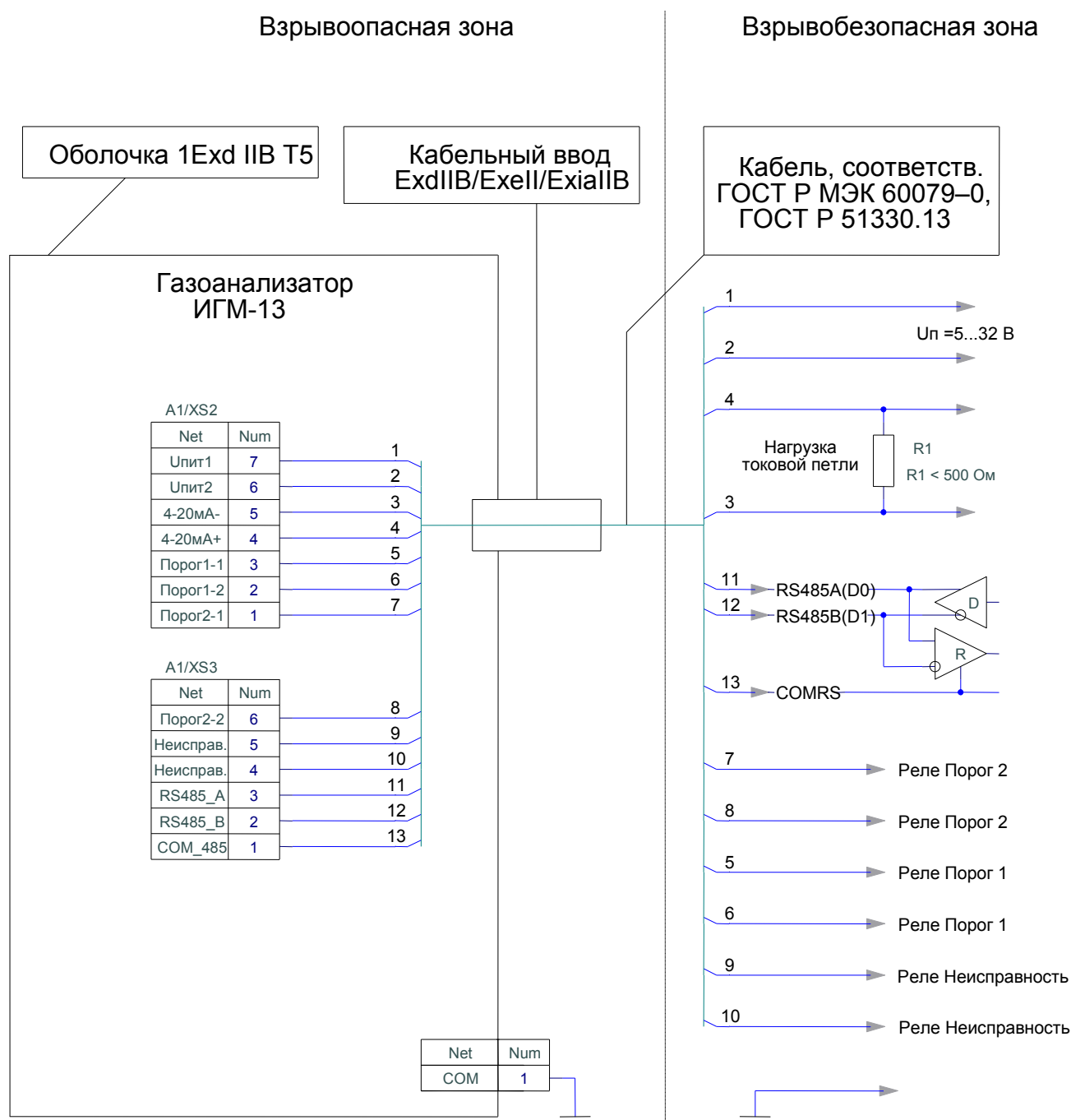
Рисунок Б.1 – Схема подключения газоанализатора ИГМ-13
